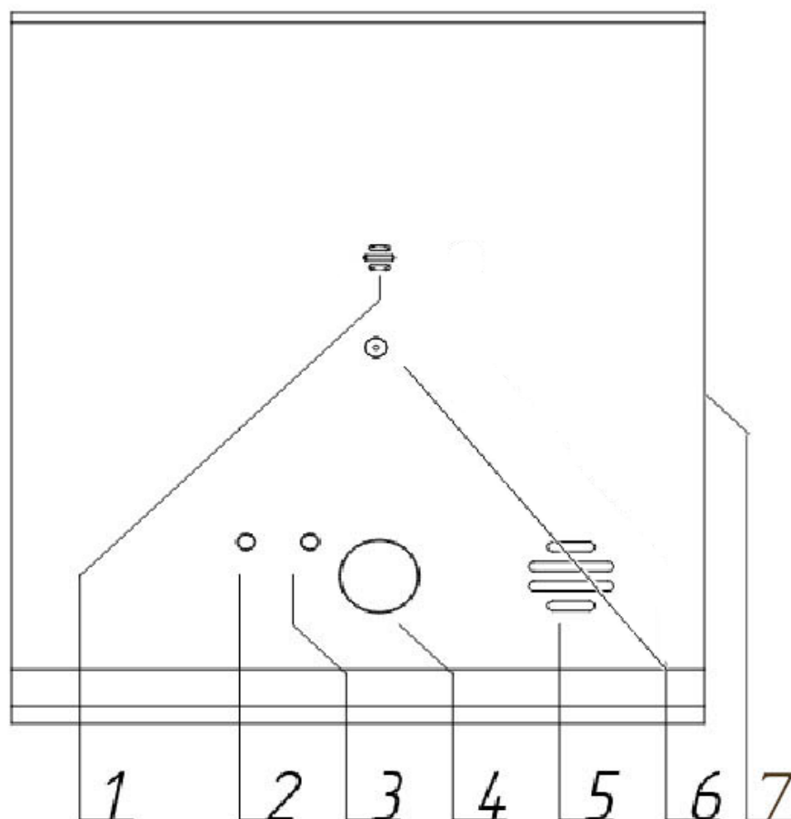
Рисунок 1 - Вызывная панель, вид спереди
