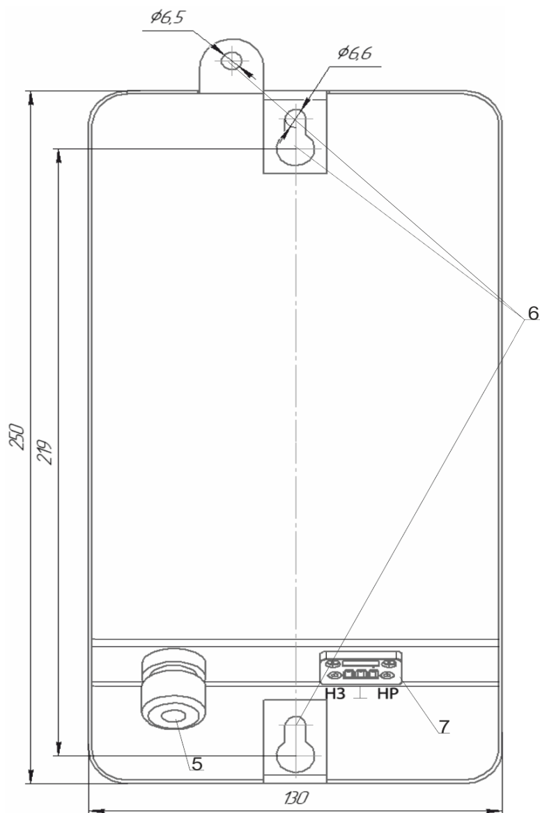
Рисунок 2 - Вид сзади
