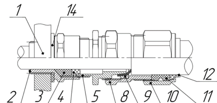
Рисунок 8 - Прокладка бронекабеля с двойным уплотнением.
