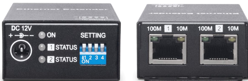
Рис.1 IP09, внешний вид спереди/сзади
