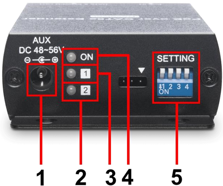
Рис. 2 IP09PT / IP09PR, разъемы и индикаторы на передней панели
