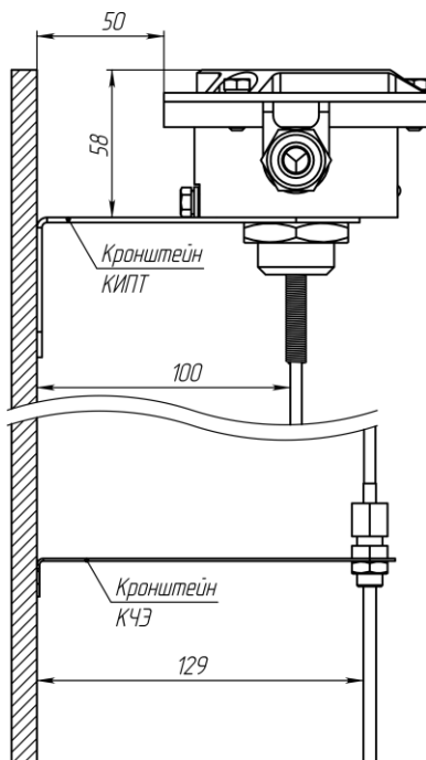
б) Крепление ИП101-07а-И2
