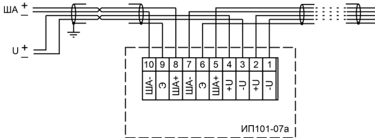
Рисунок Б.2 - Схема подключения адресных извещателей ИП101-07а в четырехпроводную адресную линию связи "ША" ППКИУП "Vesta 01F" или модуля "МС-5" с транзитом линии электропитания.
