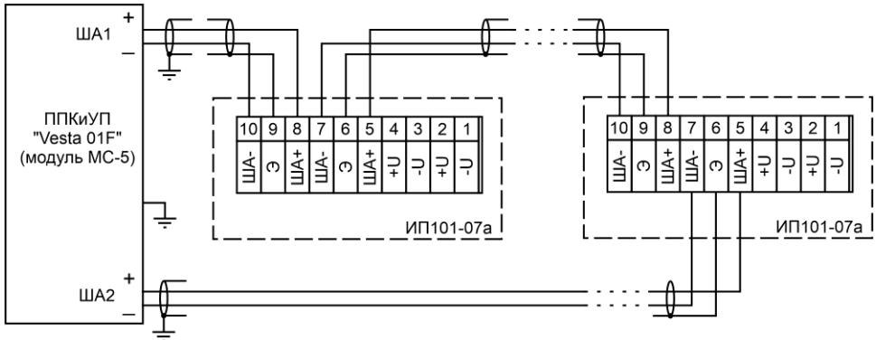
Рисунок Б.1 - Схема подключения адресных извещателей ИП101-07а в двухпроводную адресную линию связи "ША" ППКИУП "Vesta 01F" или модуля "МС-5".
