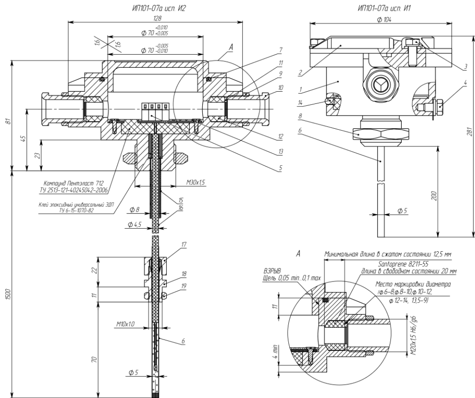
а) В корпусе из алюминиевого сплава
