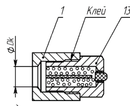
ж) монтаж оконечного элемента ОЭ
