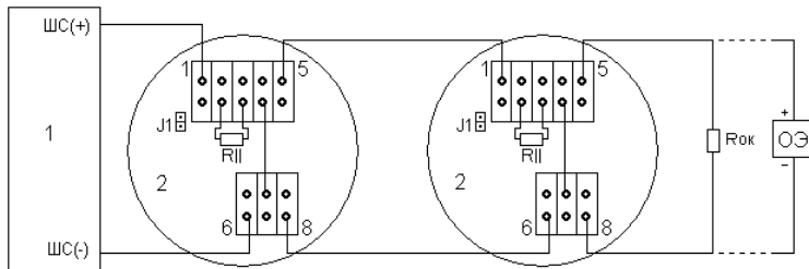
б) Схема подключения ИП101-07е на замыкание
