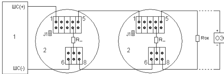
а) Схема подключения ИП101-07е на размыкание
