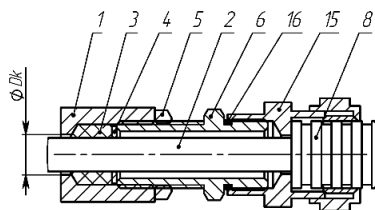
г) монтаж кабелем в металлорукаве KBМ
