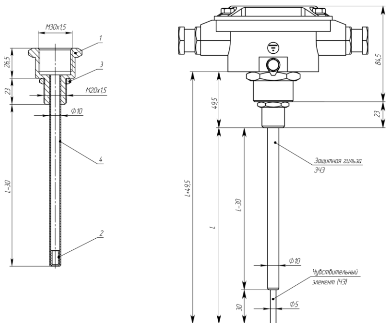
Рисунок А.3 - Монтаж защитной гильзы ЗЧЭ извещателя
