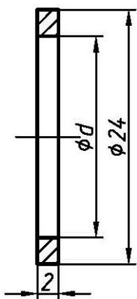
Рисунок А.21 Шайба. Материал - Сталь 20 или Д16Т. Размеры см в таблице А.8
