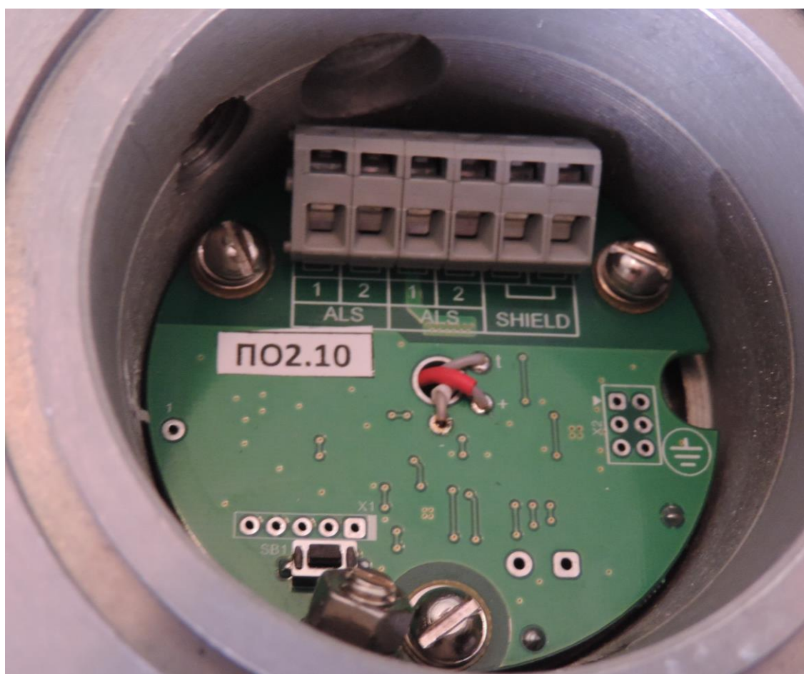
Рис. А.22 Маркировка версии программного обеспечения на плате ИП101-1В-РЗ
