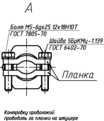
Рисунок А.11. Элементы взрывозащиты кабельного ввода для прокладки бронированного кабеля.
