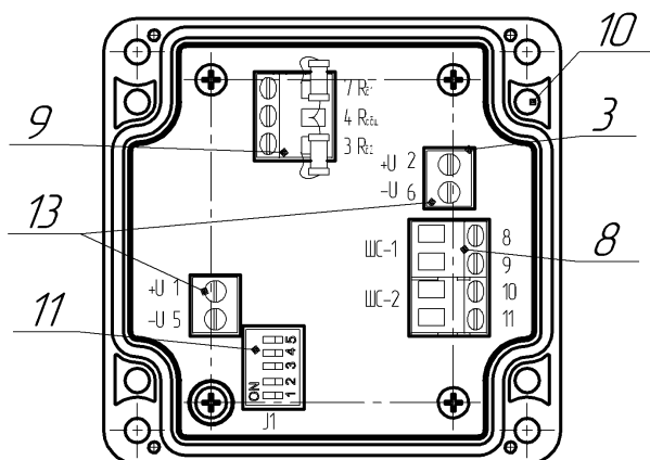
Рис. А.2. Вид со стороны подключения кабелей для модуля МИП-М-Ех.
