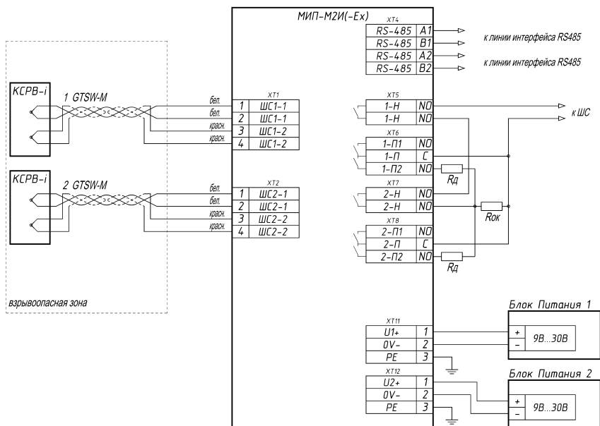
Рис. Г.2. Схема подключения модулей «МИП-М2И(-Ex)» для передачи извещений в один шлейф сигнализации.
