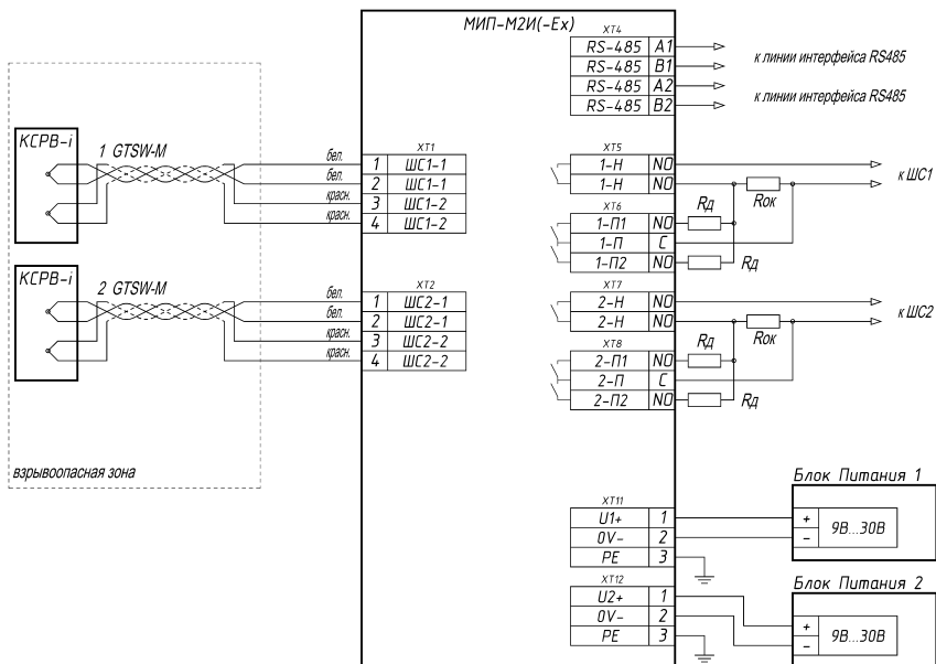
Рис. Г.1. Схема подключения модулей «МИП-М(1...2)И(-Ex)».
