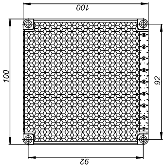
Рефлектор-отражатель ДПРМ.203625.003 (тип М) (см. табл.1)
