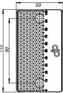
Рефлектор-отражатель ДПРМ.203625.004 (тип СМ) (см. табл.1)
