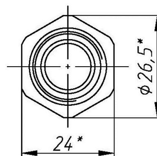
Рисунок А.8.а Штуцер для прокладки кабеля в трубе с присоединительной резьбой G1/2-B
