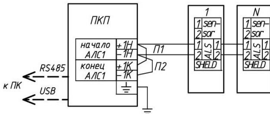
Рисунок Б.1 – Схема включения извещателей ИП212-1В-РЗ к ППКОПУ
