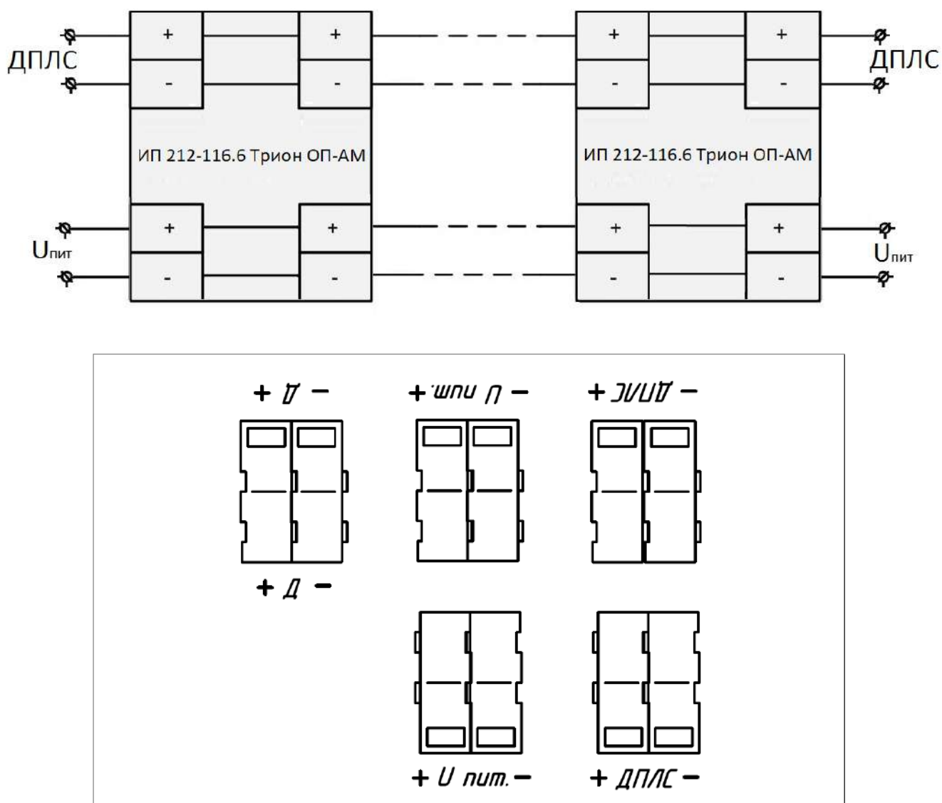
Рис. Б3 Схема подключения и расположение клемм для варианта с адресной меткой (Добавочные резисторы не требуются)
