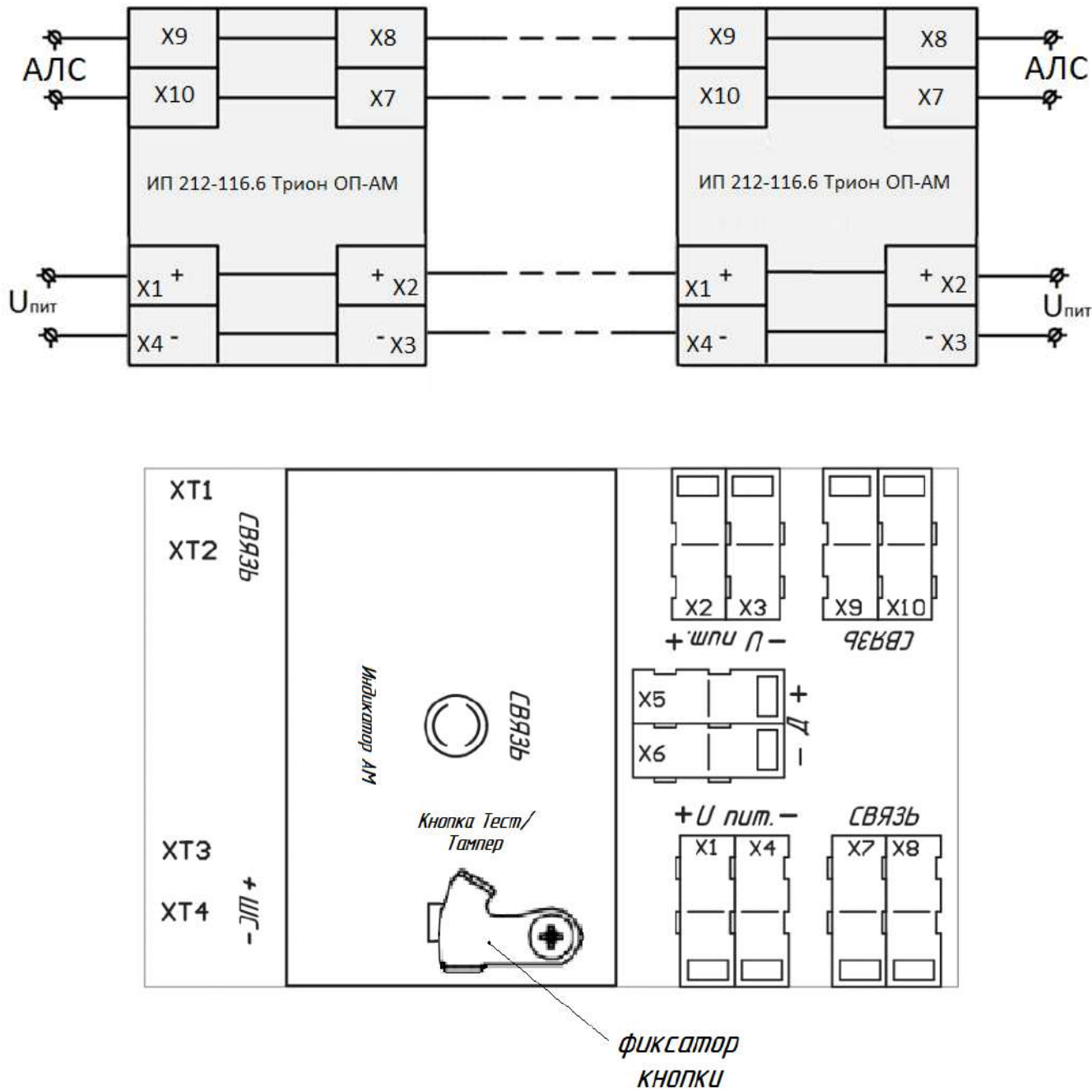
Рис. Б4 Схема подключения и расположение клемм для исполнения с адресной меткой «Рубеж» (дополнительные резисторы не требуются)
