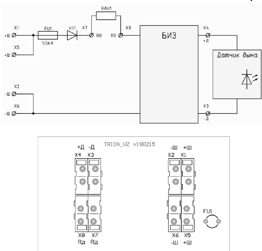
Рис. Б1 Извещатель ИП 212-116.6 Трион ОП. Схема принципиальная.
