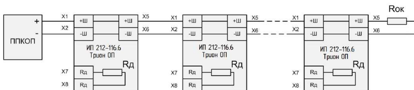
Рис. Б1 Извещатель ИП 212-116.6 Трион ОП. Схема принципиальная.
