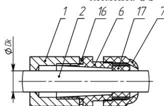
и) монтаж в кабельном вводе КВП12
