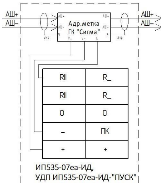
Рисунок 4 - Схема подключения адресного извещателя ИП535-07еа-ИД, адресного устройства УДП ИП535-07еа-ИД-«ПУСК» с помощью адресной метки «СИГМА» к адресному шлейфу «АШ»
