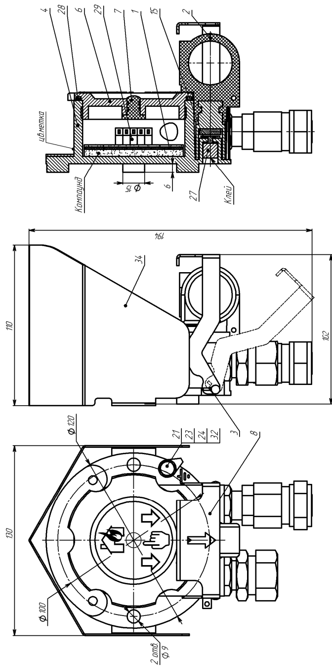
б) Внешний вид извещателя ИП535-07ea-R2-B-O
