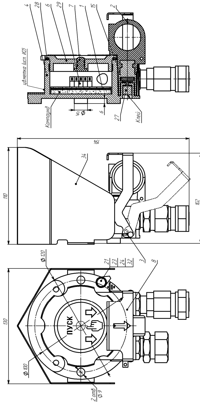
в) Внешний вид устройства ИП535-07ea-R2-“ ПУСК” -О
