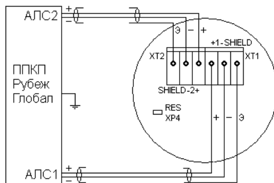
Рисунок 4. Схема подключения адресного извещателя ИП535-07ea-R2-О к двухпроводной кольцевой АЛС приборов “Рубеж-Глобал” с поддержкой протокола “RS-R2”
