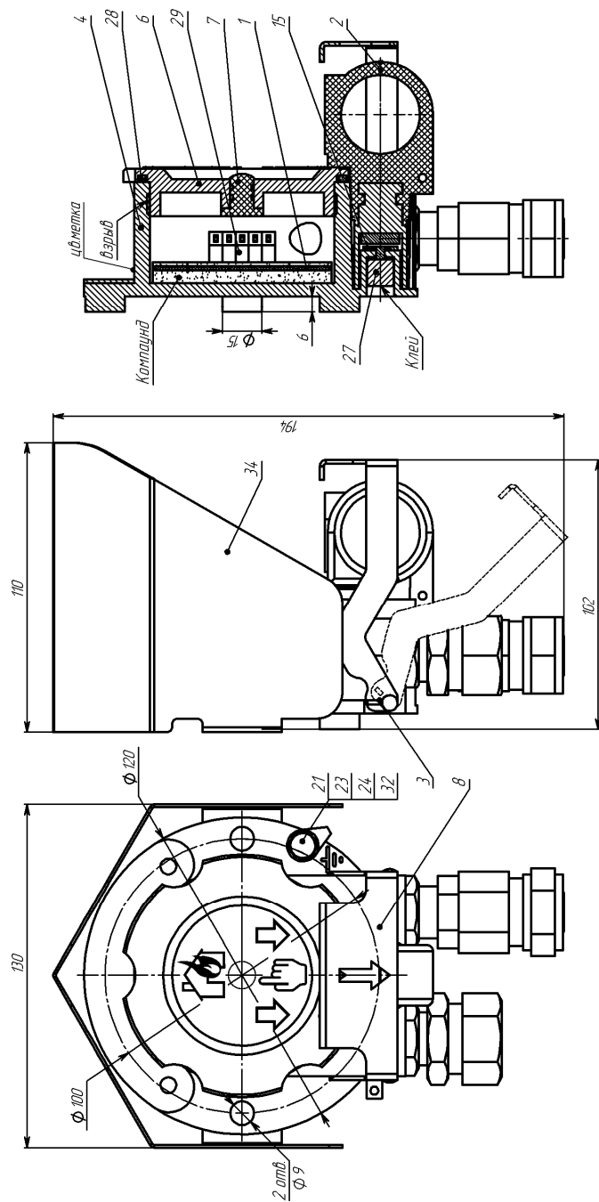
б) Внешний вид извещателя ИП1535-07са-R2-B
