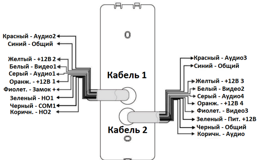
Вид сзади
