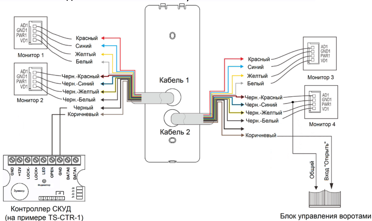
Схема 3 Подключение контроллера СКУД и блока управления воротами (управление воротами только для панели на 4 абонента).
