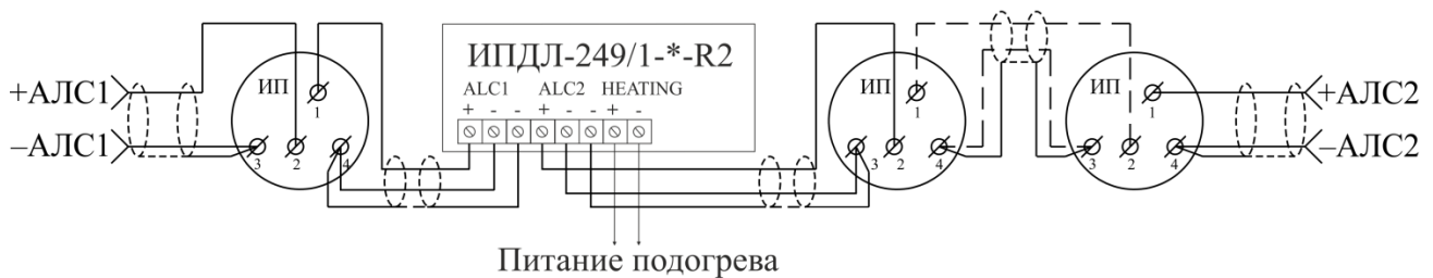
Рисунок В.2 - Схема подключения извещателей к кольцевой АЛС
