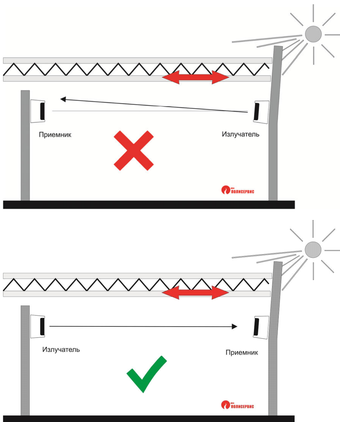
Рисунок 15: Установка ИПДЛ на стены не соединенные с капитальной конструкцией.
