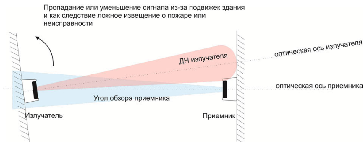
Рисунок 8: Уход луча излучателя. Выдача ложной тревоги.
