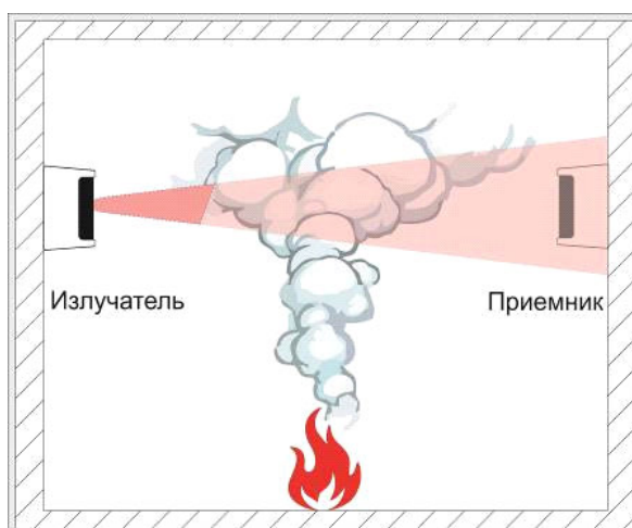
Рисунок 2: Принципиальная схема работы двухпозиционного ИПДЛ.
