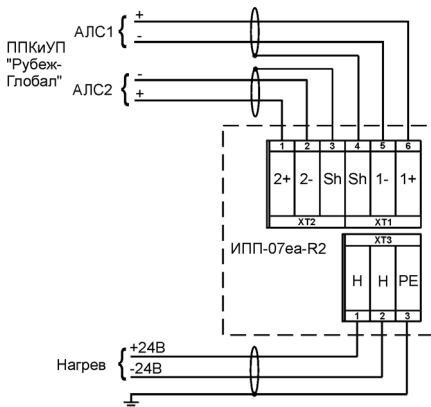
Рисунок 4. Схема подключения адресного извещателя ИПП-07еа-Р2 к двухпроводной кольцевой АЛС приборов “Рубеж-Глобал” с поддержкой протокола “RS-R2”
