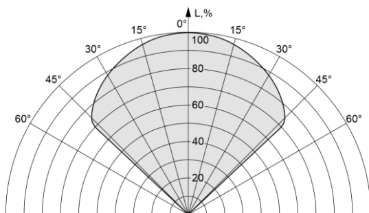
Рисунок А.5 - Диаграмма направленности ИПП-07ea-RS-HART
