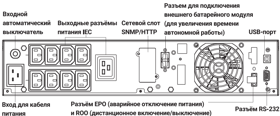
ИБП Ампер 3000
