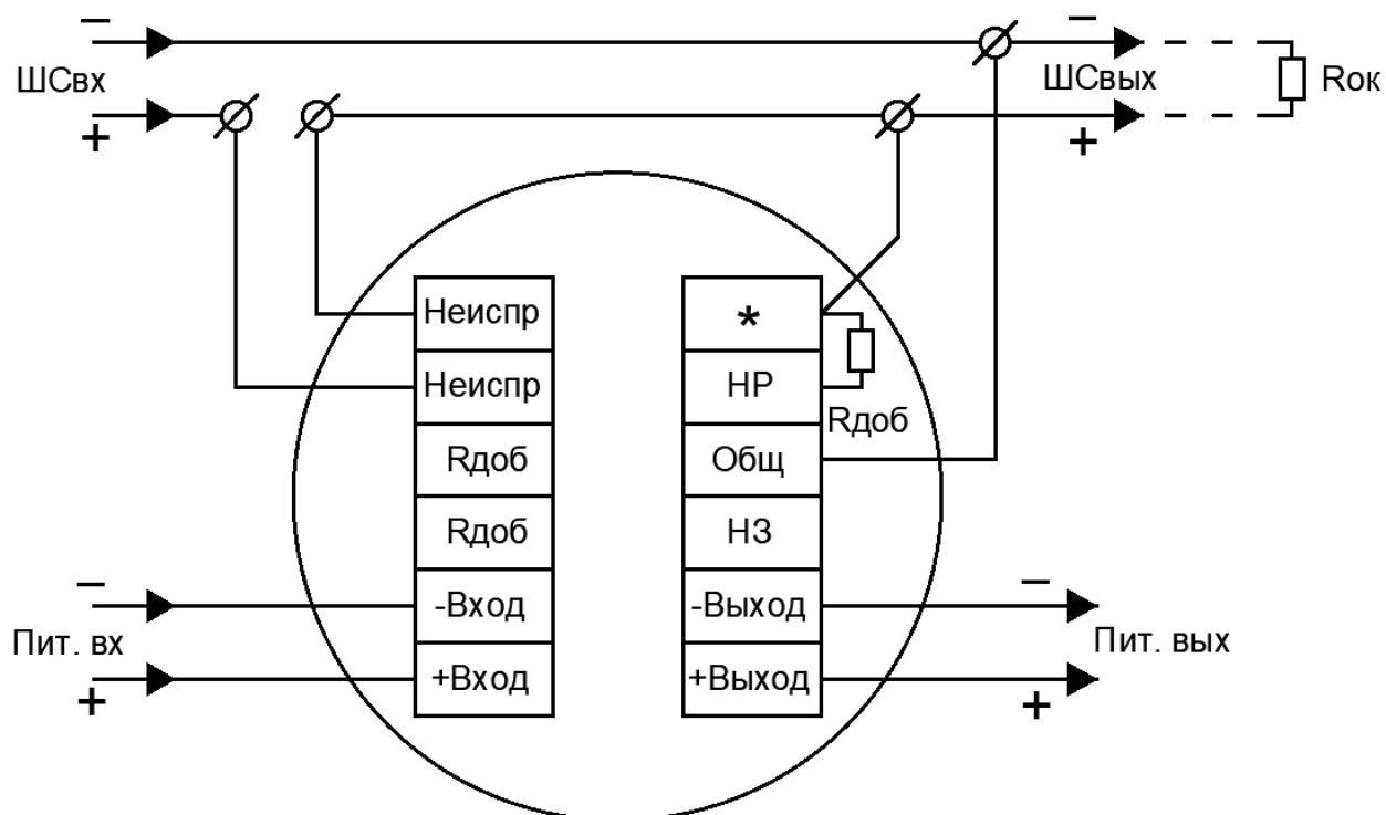
Рисунок 7 – 4-х проводная схема подключения с использованием режима неисправность
