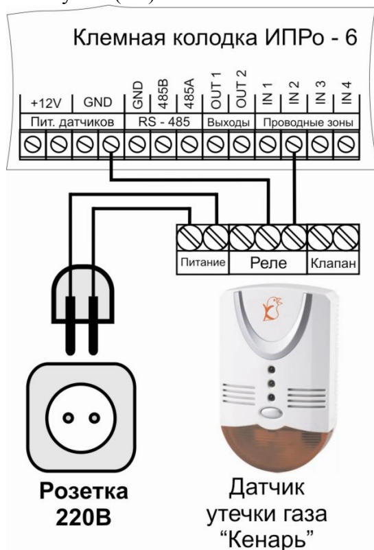
Подключение 1 датчика
