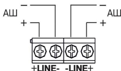
Рис. 6 Подключение проводов
