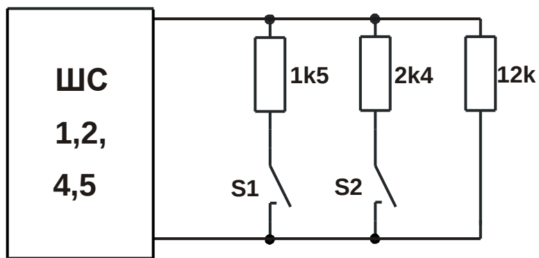
Рис. 10 Параллельное подключение 2 извещателей с НР контактами
