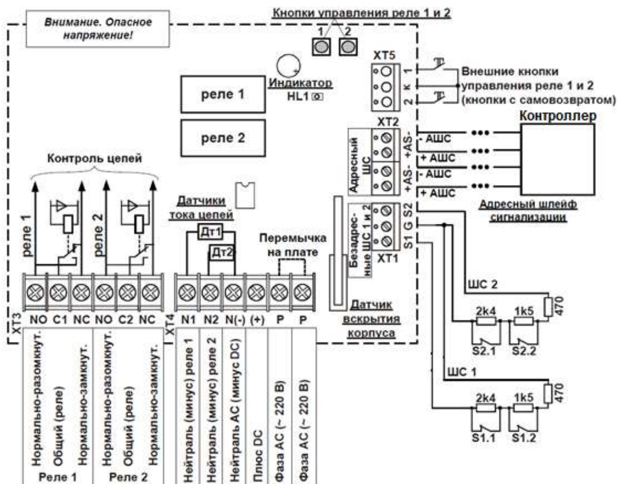
Рис. 2 Расположение элементов, подключение ИСМ220
