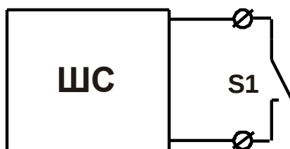
Рис. 14 Подключение извещателя с НР контактами без контроля целостности ШС
