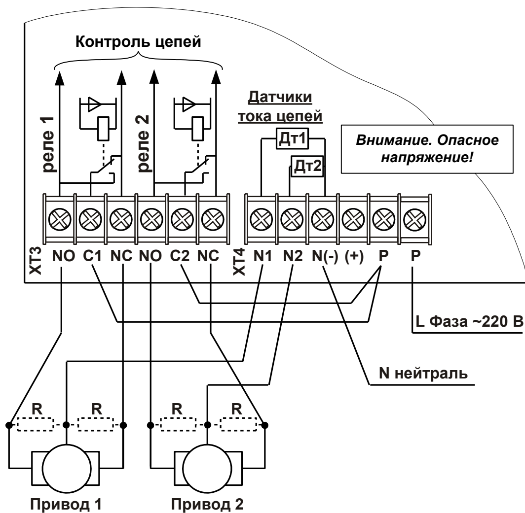
Рис. 5 Подключение двух реверсивных приводов переменного тока типа "Белимо"
