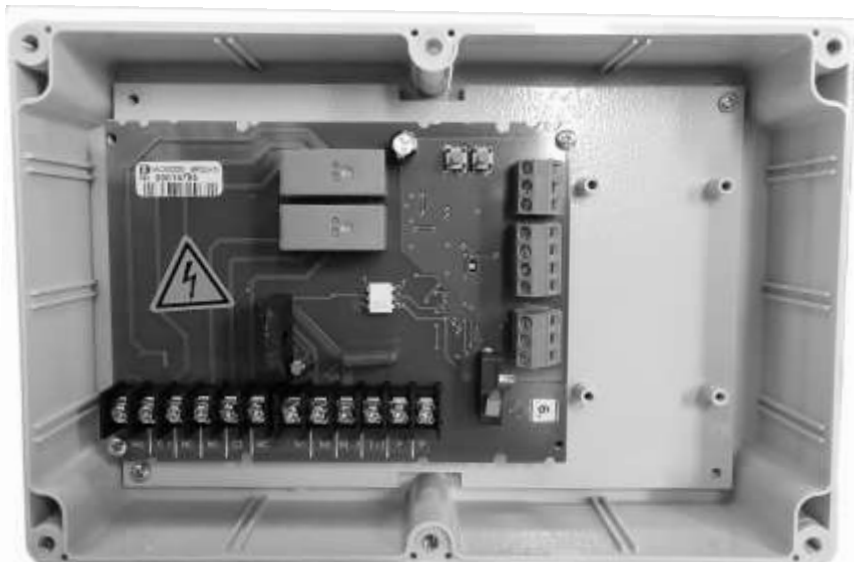
Рис. 1 Внешний вид ИСМ220 со снятой крышкой
