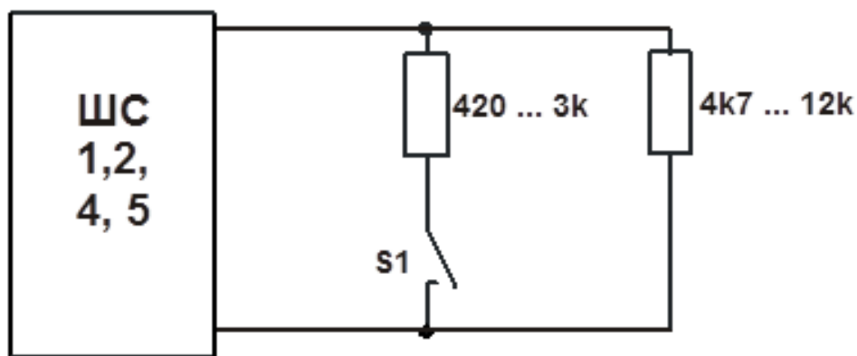
Рис. 12 Параллельное подключение 1 извещателя с НР контактами
