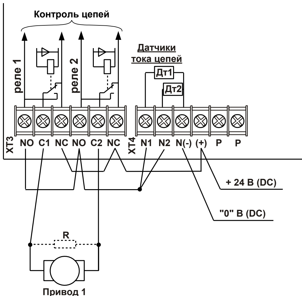
Рис. 8 Подключение реверсивного привода постоянного тока с переполюсовкой
