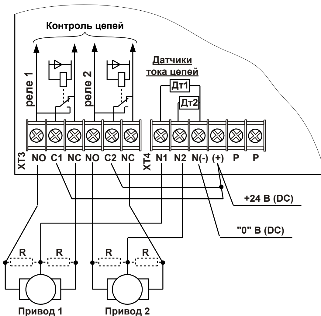
Рис. 7 Подключение двух реверсивных приводов постоянного тока типа "Белимо"
