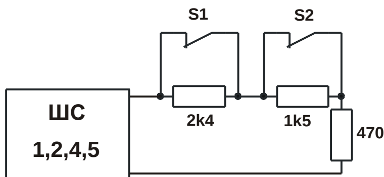
Рис. 9 Последовательное подключение 2 извещателей с НЗ контактами
