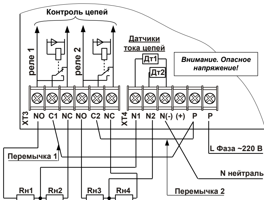
а) Подключение нагрузок к сети переменного тока ~220 В, 50 Гц, ~U - (160 ... 260) В, I_n \leq 3 А
