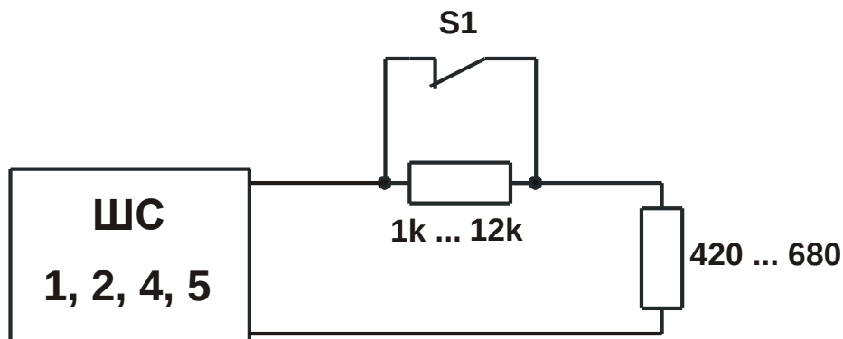
Рис. 11 Последовательное подключение 1 извещателя с НЗ контактами
