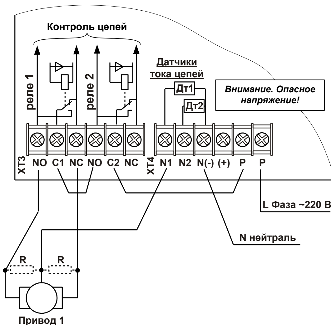
Рис. 6 Подключение одного реверсивного привода переменного тока типа "Белимо" с возможностью отключения напряжения
