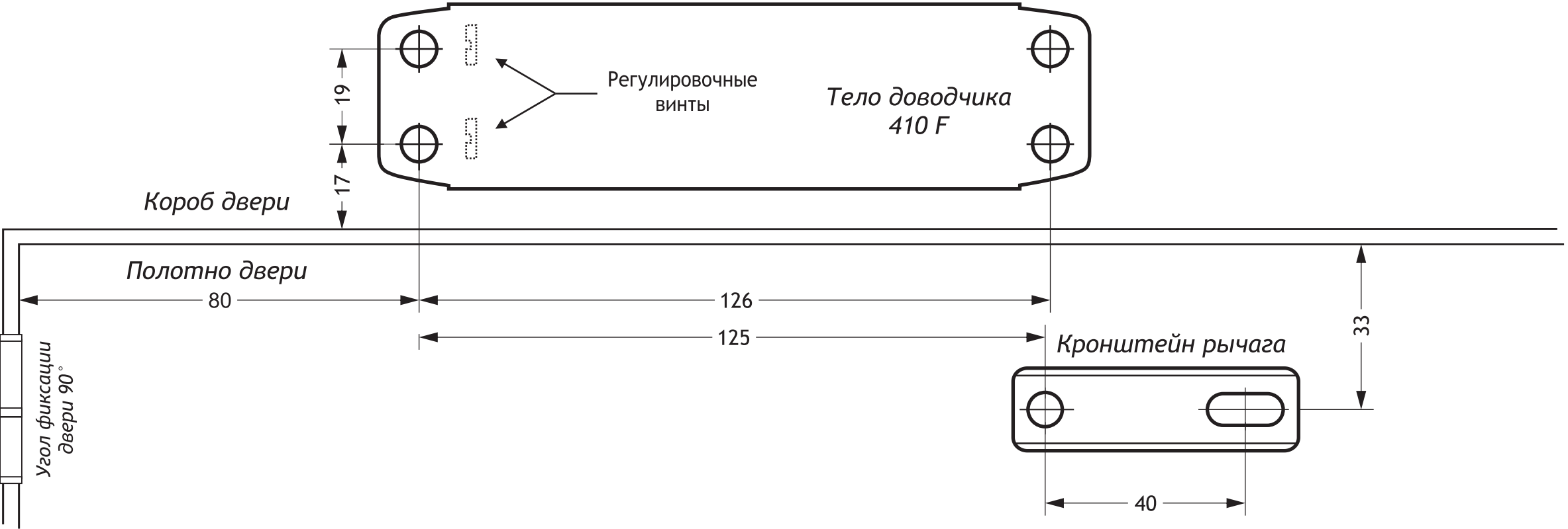
Шаблон установки на короб левой двери
