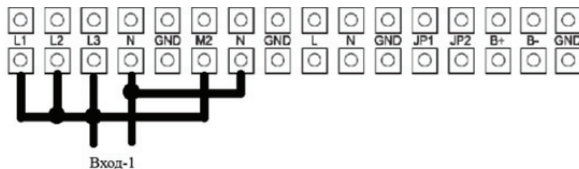
Рис. 4-7-б Схема подключения при однофазном входе и одной питающей линии
