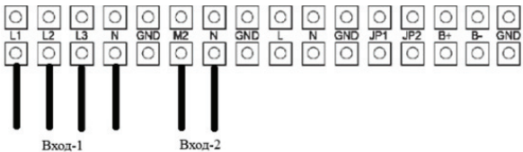
Рис. 4-б-в Схема подключения при трехфазном входе и раздельных питающих линиях
