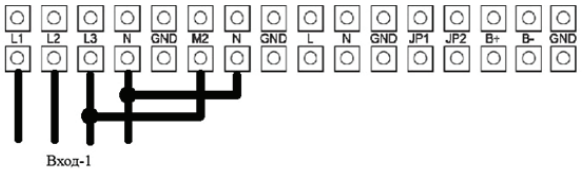
Рис. 4-б-г Схема подключения при трехфазном входе и одной питающей линии
