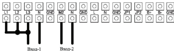
Рис. 4-7-а Схема подключения при однофазном входе и раздельных питающих линиях
