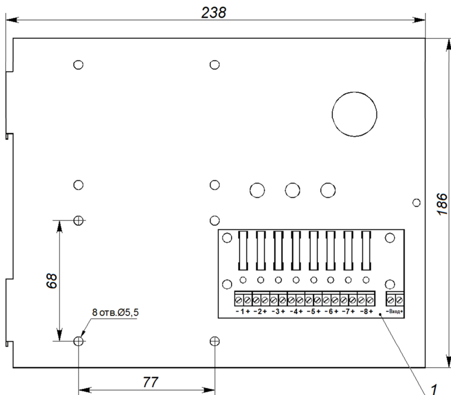
1 - модуль УРП-1-8
