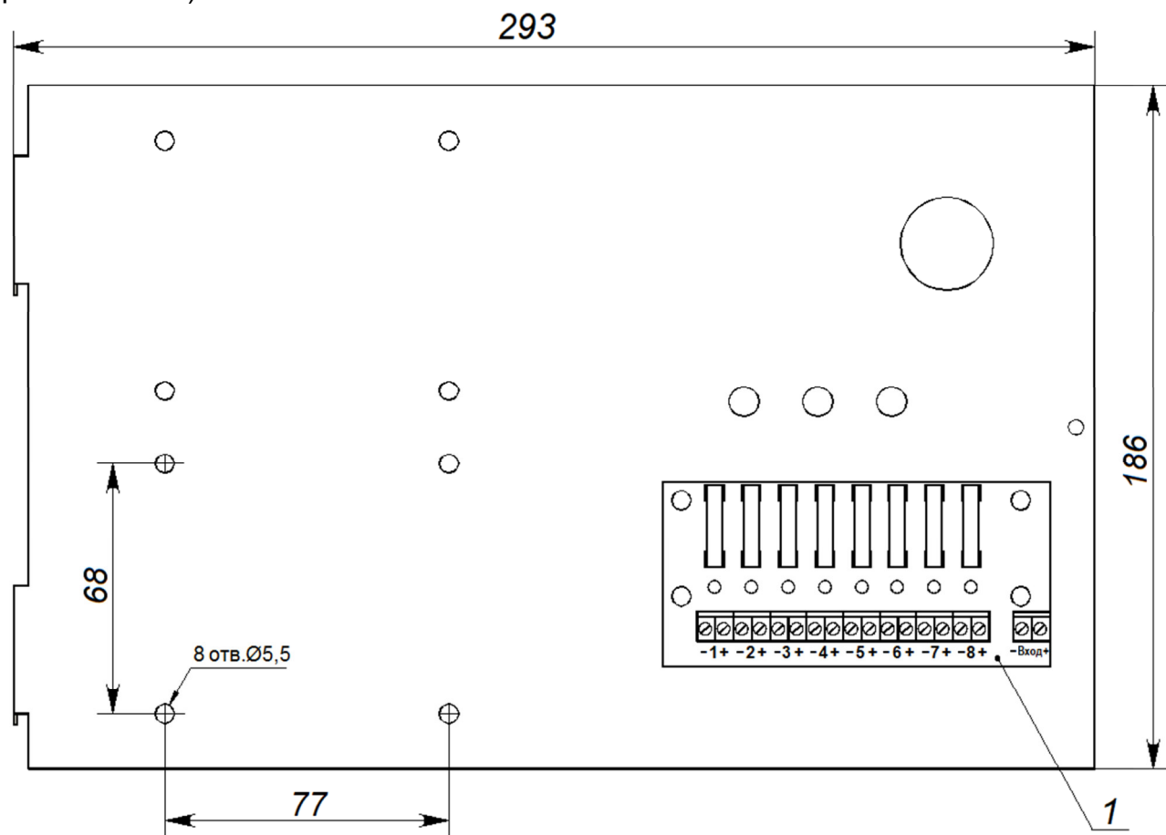
1 - модуль УРП-1-8
