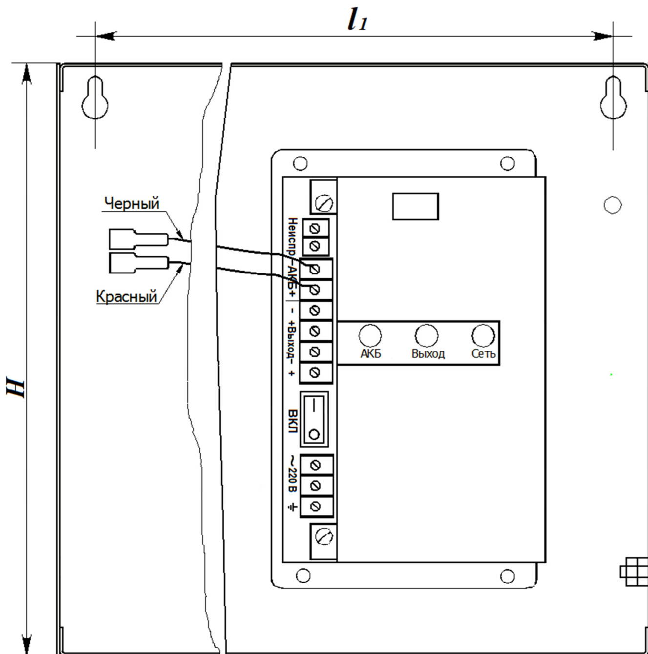
Рисунок 1 - Общий вид БРП со снятой крышкой
