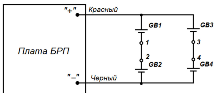
а) Схема соединения двух АКБ с платой БРП
