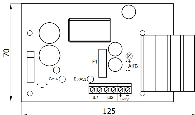
Рисунок 2 - Общий вид платы БРП1
