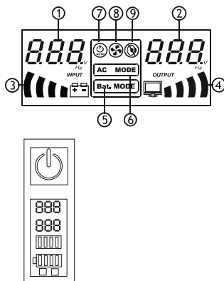
Рисунок 2 – Дисплей ИБП серии ELACTRA ET
