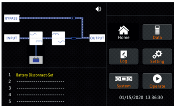
Рисунок 28 – Экран запуска инвертора
