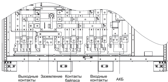
Рисунок 22 – Шина с клеммами для моделей 250–300 кВА
