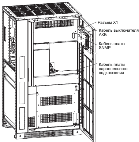
Рисунок 33 – Сигнальные кабели ИБП 100–600 кВА
