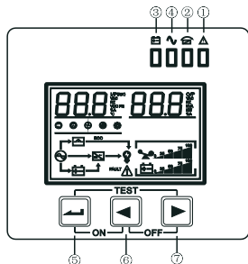
Рисунок 6 – Панель управления
