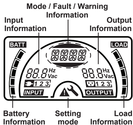
Рисунок 4.2 LCD дисплей
