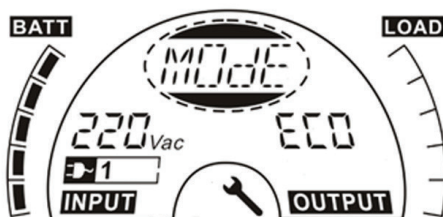
Шаг 5: “ECO” мигает после нажатия кнопки Выбор.
