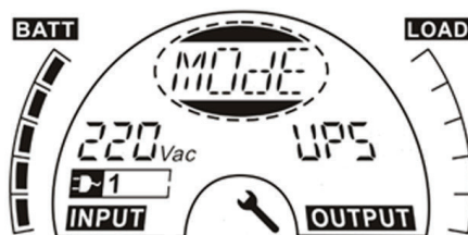
Шаг 4: “MOdE” после нажатия кнопки Выбор. “UPS” мигает после нажатия кнопки Ввод.
