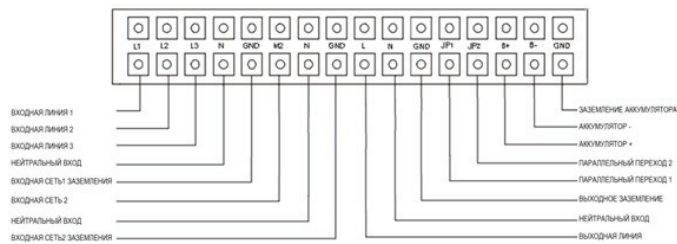
Рис. 4-6-а Схема проводки для блока контактов ввода и вывода
