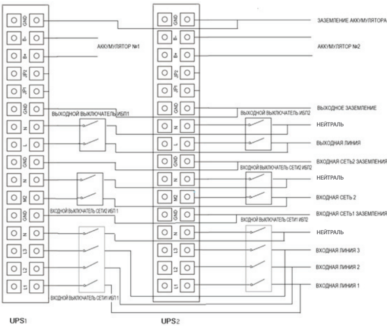
Рис. 6-1 Схема проводки для блока контактов ввода и вывода для моделей 10 кВА / 20 кВА
