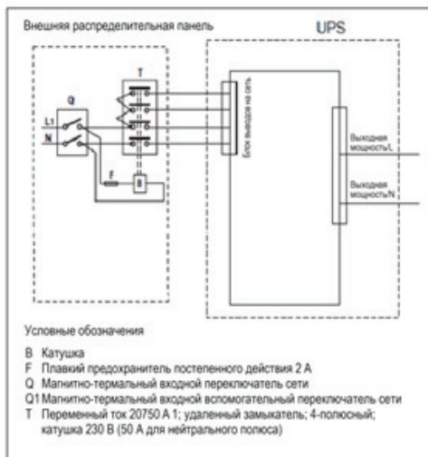
Рис. 6-5 Модель 10 кВА Компакт и внешнее изолирующее устройство
