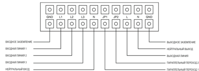
Рис. 4-6-б Схема проводки для блока контактов ввода и вывода
