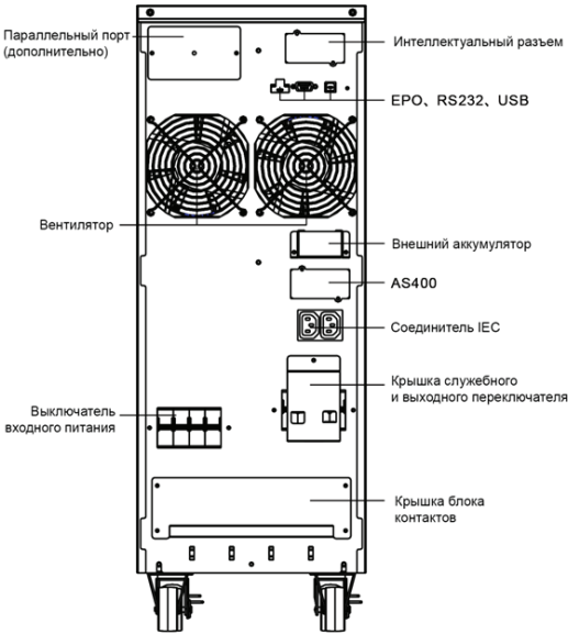
Рис. 3-1 Вид сзади линейки трехфазных ИБП
