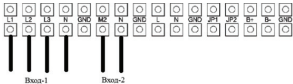
Рис. 4-6-в Схема подключения при трехфазном входе и раздельных питающих линиях
