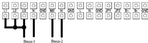
Рис. 4-7-а Схема подключения при однофазном входе и раздельных питающих линиях
