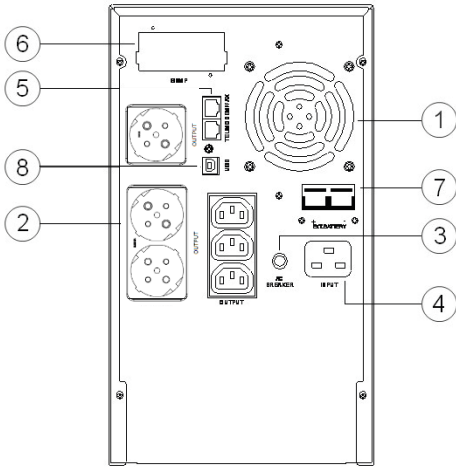
Исполнение Tower модели 1000 – 2000 ВА (слева) и 3000 ВА (справа)
