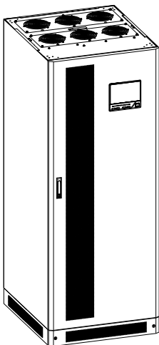
Рисунок 3 – Внешний вид ИБП типа МРОВ-100-3-00-Т, МРОВ-120-3-00-Т, МРОВ-160-3-00-Т, МРОВ-200-3-00-Т / Figure 3 – UPS appearance of МРОВ-100-3-00-Т, МРОВ-120-3-00-Т, МРОВ-160-3-00-Т, МРОВ-200-3-00-Т types
