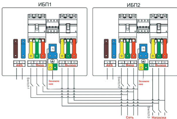
Рисунок 112 – Схема подключения ИБП типа МРОВ130 мощностью 40 кВА – 80 кВА в параллельную систему, конфигурация 33 с общим входом
