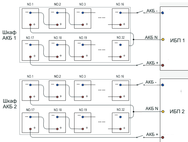
Рисунок 84 – Схема подключения двух шкафов АКБ для ИБП типа МРОВ120/121
