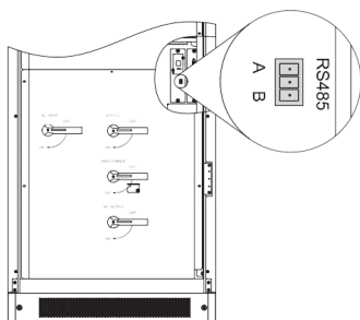
Рисунок 126 – Расположение порта RS 485 ИБП типа МРОВ230 мощностью 100 кВА – 200 кВА
