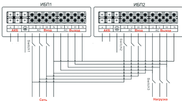
Рисунок 111 – Схема подключения ИБП типа МРОВ130 мощностью 10 кВА – 30 кВА в параллельную систему, конфигурация 33
