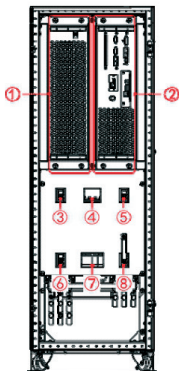
Рисунок 10 – Расположение основных элементов ИБП типа МРОВ130 мощностью 60–120 кВА (дверь открыта)
