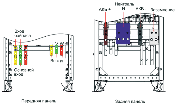
Рисунок 86 – Схема подключения для ИБП типа МРОВ130 мощностью 60–120 кВА
