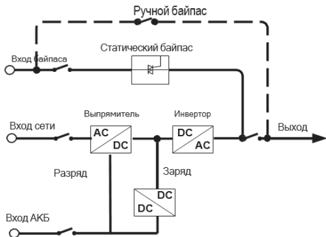
Рисунок 26 – Схема ИБП
