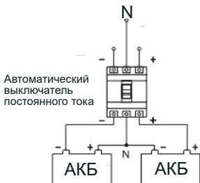
Рисунок 23 – Схема подключения АКБ
