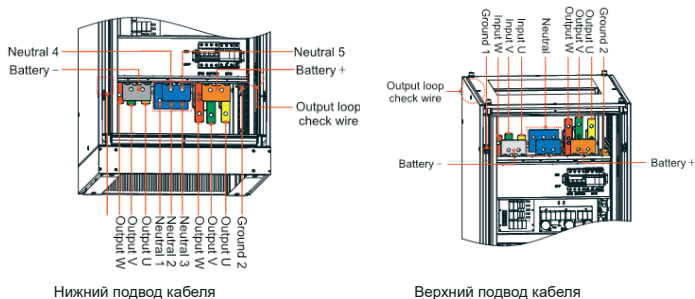
Рисунок 22 – Подключение кабелей
