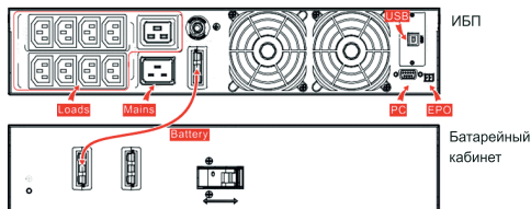
Рисунок 60 – Схема подключения ИБП типа MPOR111 мощности 2 кВА / 3 кВА к батарейному кабинету
