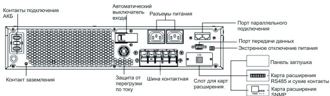
Рисунок 17 – Внешний вид задней панели ИБП типа MPOR110
