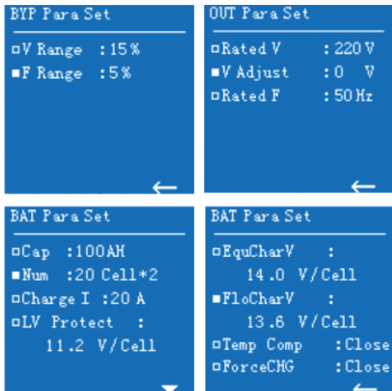
Рисунок 50 – Страницы параметров ИБП
