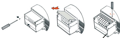
Рисунок 71 – Демонтаж защитной крышки контактов ИБП типа MPOR120
