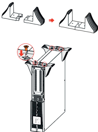
Рисунок 22 – Крепление опор на корпус ИБП
