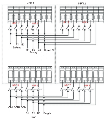
Рисунок 78 – Подключение ИБП типа MPOR120 мощностью 30 кВА – 40 кВА в параллельную систему, конфигурация 33
