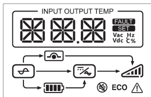
Рисунок 13 – Экран ПУ
