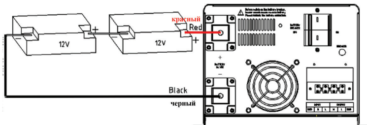
Схема подключения аккумуляторных батарей U=24В . Модель PSW-HW PROxima 2500 – 3500 Вт
