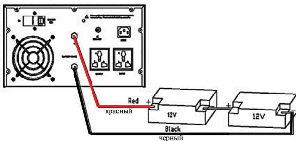
Схема подключения аккумуляторных батарей U=24В . Модель PSW-H PROxima 1600 Вт
