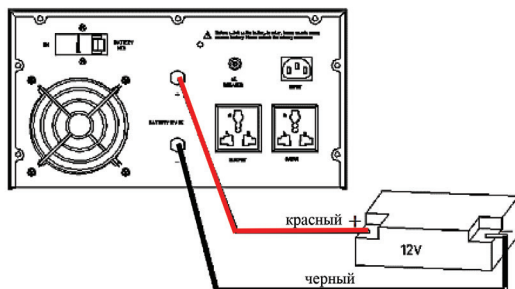
Схема подключения аккумуляторных батарей U=12В . Модель PSW-H PROxima 300 Вт – 1000 Вт
