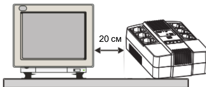
Рисунок 3-2. Подключение нагрузки
