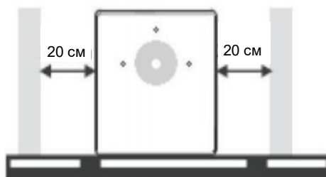
Рисунок 3-1. Установка ИБП
